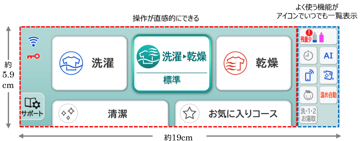
図1：ホーム画面
